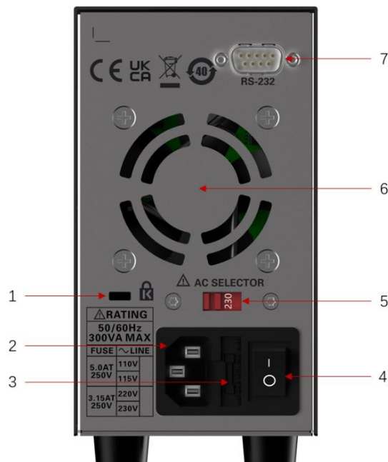
图 4.4 后面板示图
