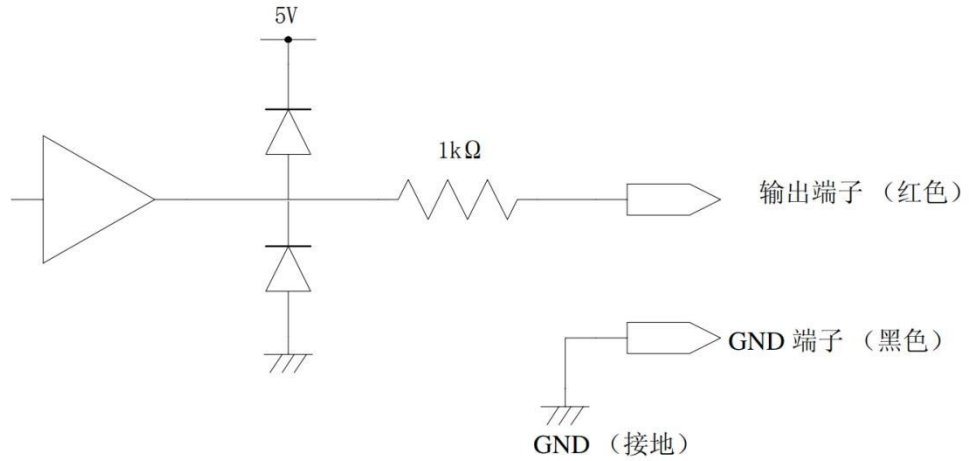
图 8.1 连接图
